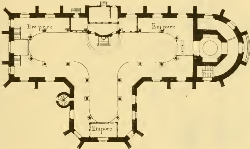
Fig. 129. Kirche zu Grossenhain, Grundriß.
